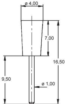
Serie / Type 239 mit Isolation / with insulation
