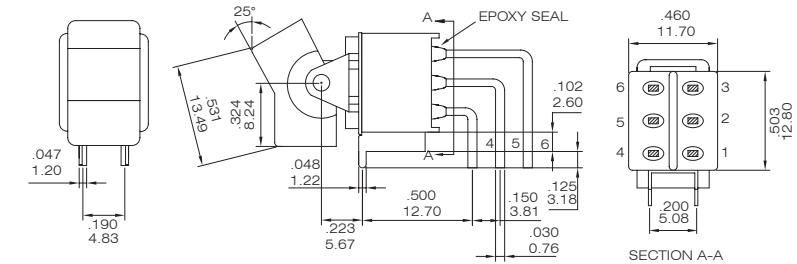
NER8011L - R11-2-Q
