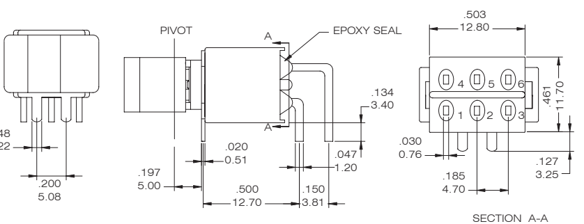
NER8017P - R11-2-Q
