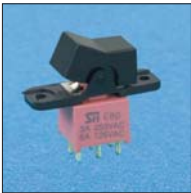
DPDT 2 Comm 1 3 4 6
