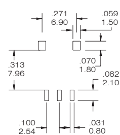
ER-3-A*-N
